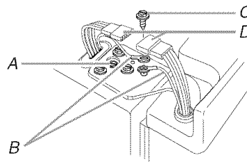
A. Ne pas enlever la vis A B. Fils de liaison à la terre C. Vis verte de liaison à la terre D. Fiche des fils
