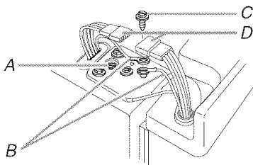
A. Ne pas enlever la vis A B. Fils de liaison à la terre C. Vis verte de liaison à la terre D. Fiche des fils
