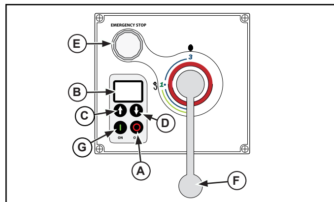
Figure 8. Panneau de commande du mélangeur 60 qt (66 l).
