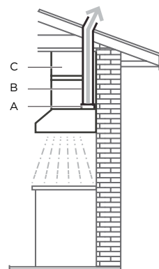
A. Transición redonda de 10" (25.4 cm) B. Conducto de 10" (25.4 cm) C. Gabinete
