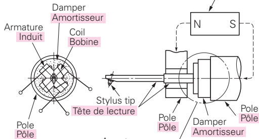
Fig. 4 Construction Sketch Fig. 4 Schéma de construction
