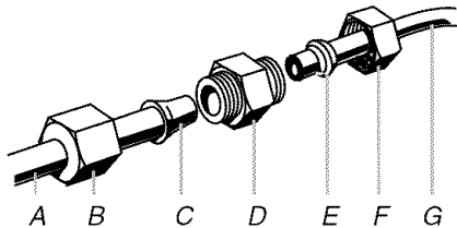
A. Tube vers le réfrigérateur D. Raccord (fourni) B. Écrou (fourni) E. Virole (à acheter) C. Renflement F. Écrou (à acheter) G. Tube vers la machine à glaçons
