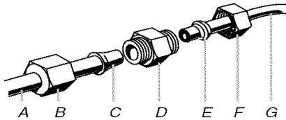
A. Tubería de agua B. Tuerca (provista) C. Bulbo D. Acoplamiento (provisto) E. Fécula (adquirida) F. Tuerca (adquirida)
