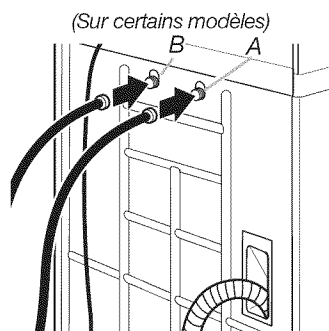
A. Électrovanne d'alimentation – eau froide B. Électrovanne d'alimentation – eau chaude
