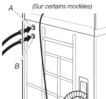
A. Électrovanne d'alimentation – eau froide B. Électrovanne d'alimentation – eau chaude
