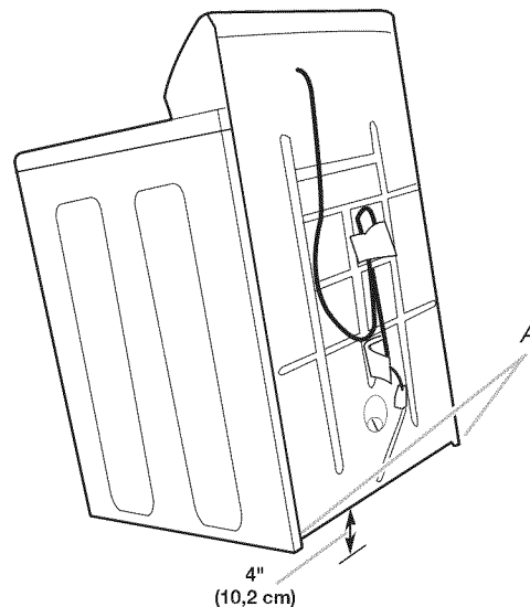
A. Pieds autoréglables
