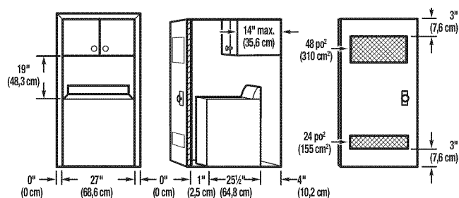
A. Vue avant
