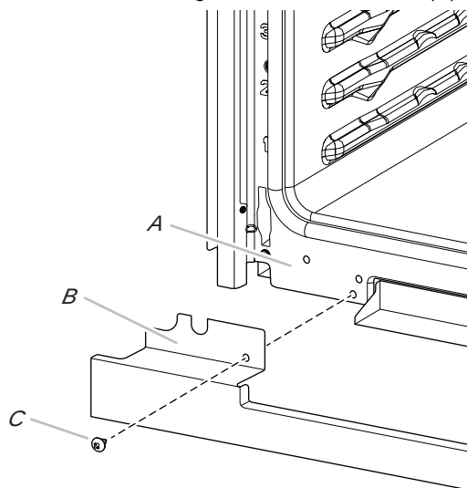
A. Marco del horno B. Lengüeta del protector C. Tornillo n.º 8-18 x 3/8" (9,5 mm)
