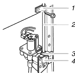
1. Bride du tube 3. Écrou de compression 2. Tube en cuivre 4. Valve d'entrée d'eau
