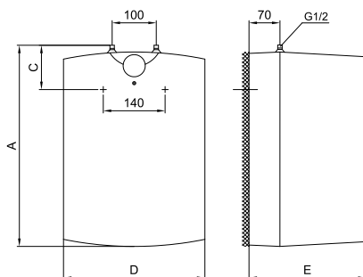
Podumivalniška izvedba
