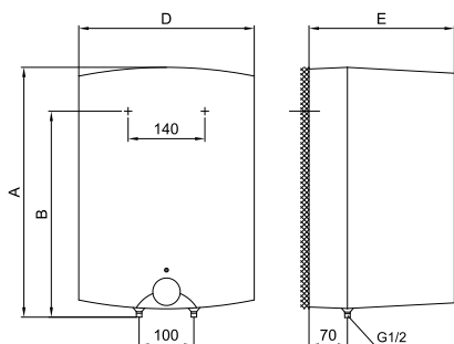
Nadumivalniška izvedba
