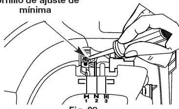
Tornillo de ajuste de mínima
