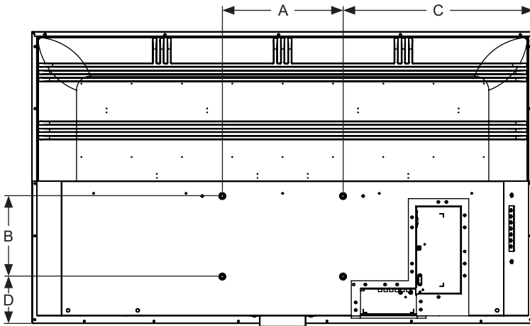
VISTA TRASERA
