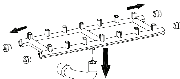
PULVÉRISATEUR D'EAU ET CAPUCHONS EN CAOUTCHOUC
