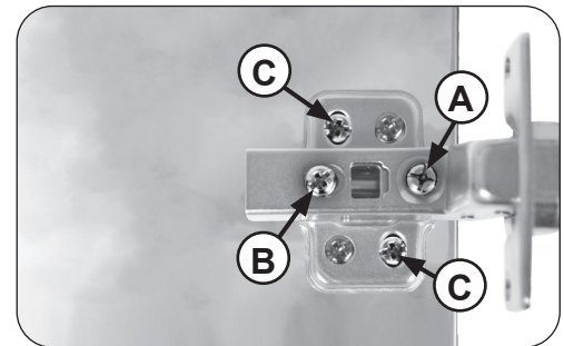
Fig. 4-2 Adjust door
