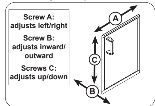
Fig. 4-3 Adjust door
