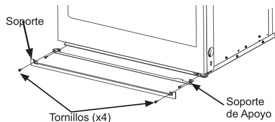
Instalación de Hornos Simples y Dobles de Pared sin Pedestal
