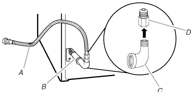
A. Connecteur à gaz souple de \frac{3}{8} " B. Conduit de la sécheuse de \frac{3}{8} " C. Coude de conduit de \frac{3}{8} " à \frac{3}{8} " D. Adaptateur entre le conduit et le joint conique de \frac{3}{8} "
