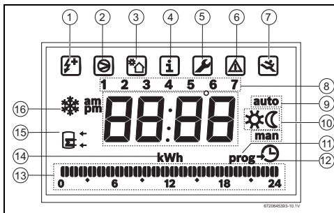
Fig. 21 Display
