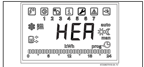
Fig. 44 „HEA“ function
