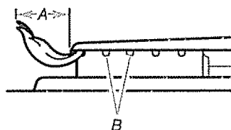
A. 1-1 1/2" (25-38 mm) B. Orificios del quemador
