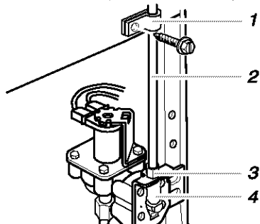
1. Bride du tube 2. Tube en cuivre 3. Écrou de compression 4. Entrée d'eau de la valve
