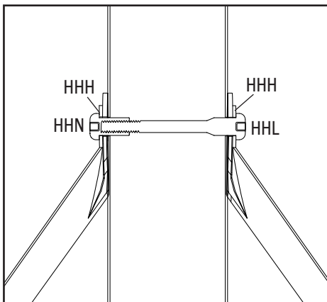
Cross section / Section transversale / Sección transversale
