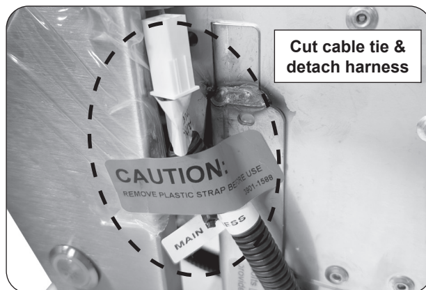
Fig. 28-3 Cut cable-tie
