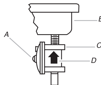
A. Chapeau de l'ouverture d'accès B. Arrière de la table de cuisson C. Détendeur D. Sens de circulation
