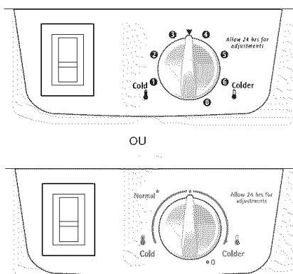
Commandes du réfrigérateur (certains modèles)
