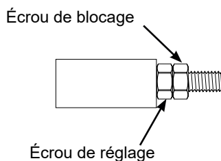
Ensemble tendeur moteur
