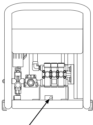
Tensor del motor
