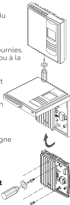
Installation à 4 fils
