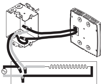
Installation à 2 fils
