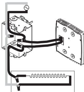
Installation à 4 fils
