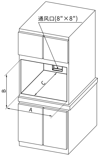
半嵌开孔示意图
