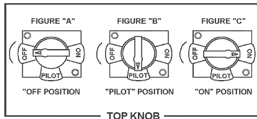
TOP KNOB
