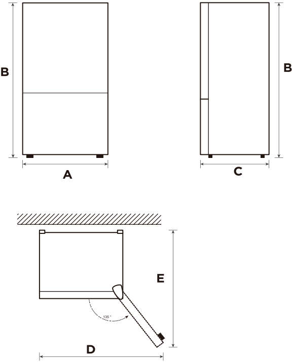
Diagram potrebnega prostora (ko so vrata odprta in ko so vrata zaprta)
