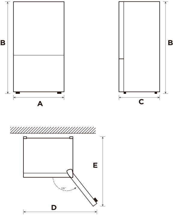
Platzbedarfsdiagramm (bei geöffneter und geschlossener Tür)
