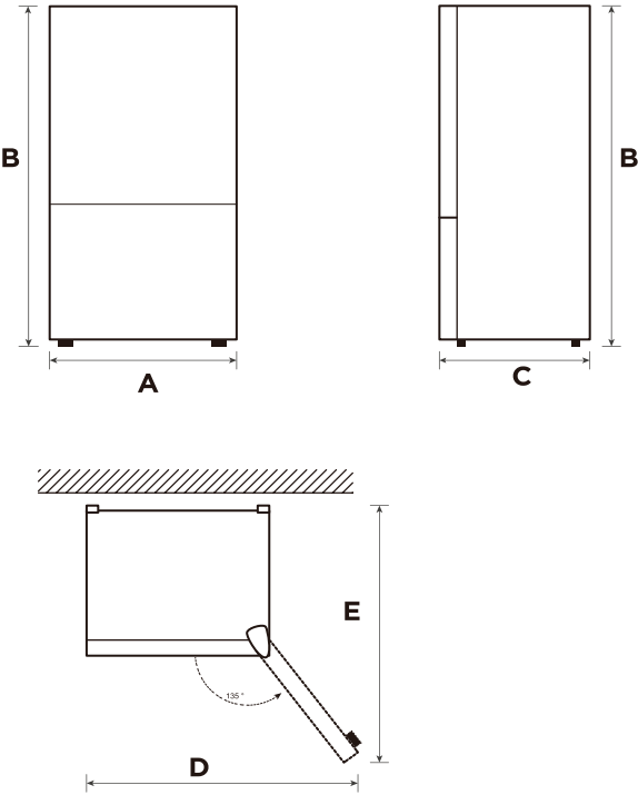
Erdvės reikalavimų diagrama (kai durelės atidarytos ir kai durelės uždarytos)
