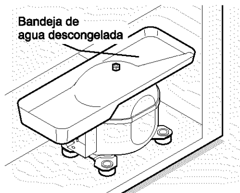
Bandeja de agua descongelada, no desmontable (en ciertos modelos)
