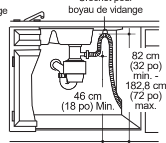
Installation avec broyeur à déchets
