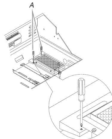
A. 2 screws
