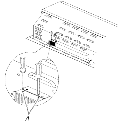
A. 2 vis
