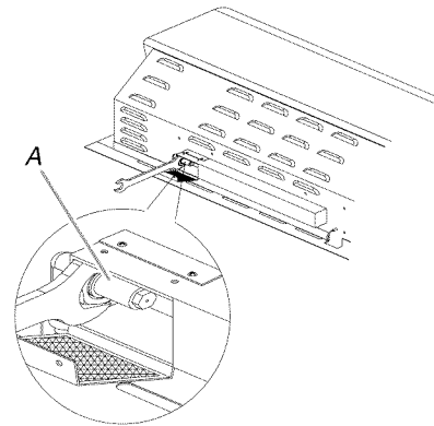
A. Écrou pour gicleur
