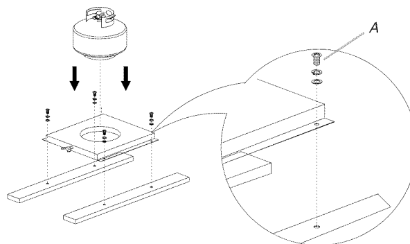
A. Cuatro tornillos de cabeza segmentada de \frac{3}{32} " x 10 mm
