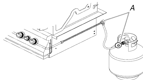
A. Ensemble détendeur/tuyau
