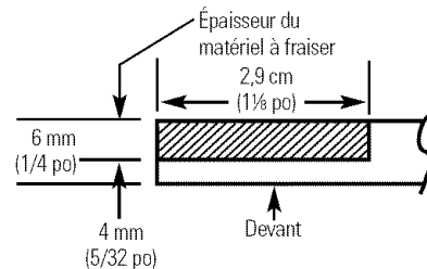
Exemple de fraissage
