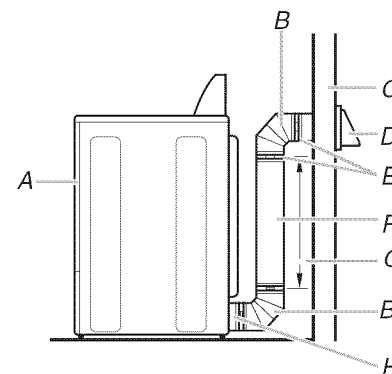
A. Sècheuse B. Coude C. Mur D. Clapet de décharge E. Brides
