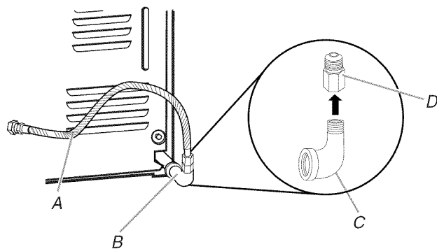
A. Connecteur de gaz souple de \frac{3}{8} " B. Conduit de la sècheuse de \frac{3}{8} " C. Coude de conduit de \frac{3}{8} " par \frac{3}{8} " D. Adaptateur entre le conduit et le joint conique de \frac{3}{8} "
