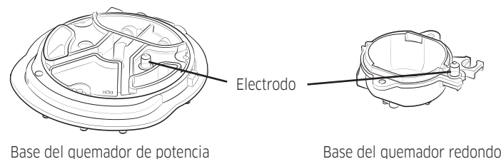
Base del quemador de potencia
