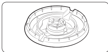
Tête des brûleurs en laiton (Uniquement pour NA30N7755T*/NA36N7755T*)
