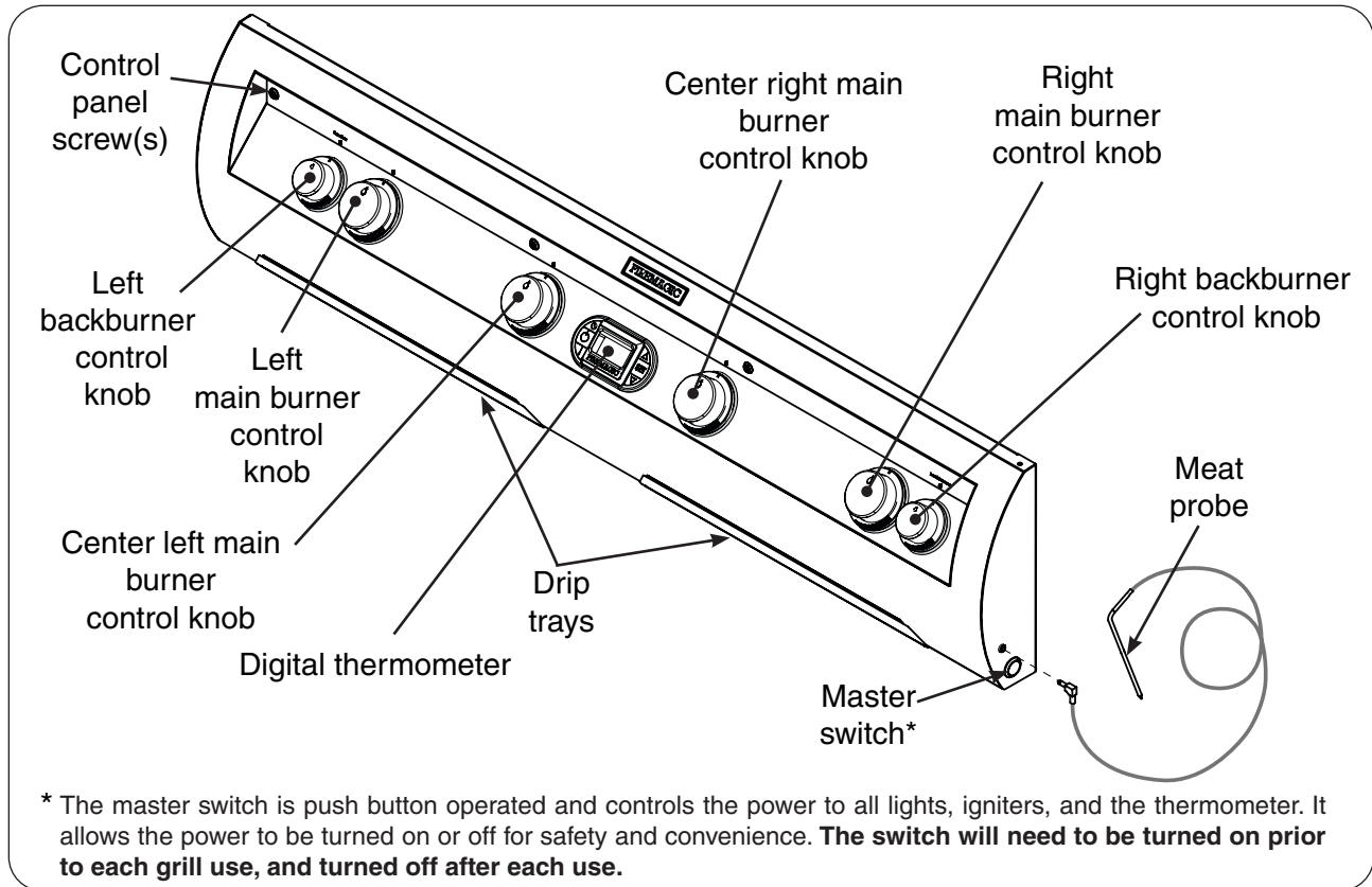
Fig. 26-1 E1060i controls
