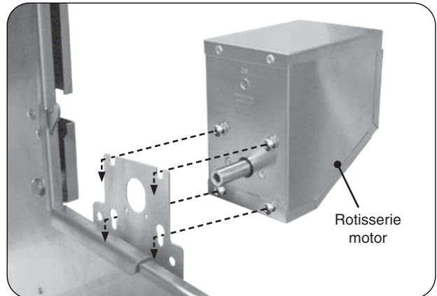
Fig. 33-2 Install rotisserie motor
