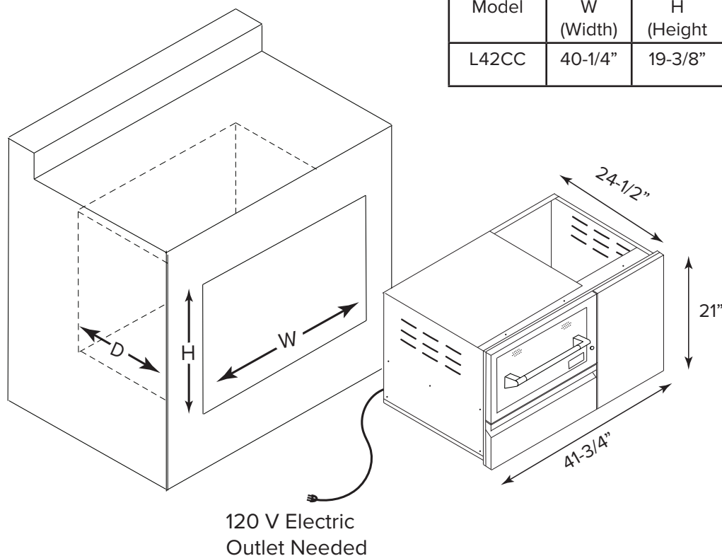
Cutout Dimensions
