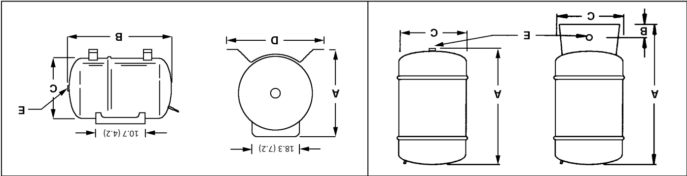
Figure 2. Dimensiones aproximadas
