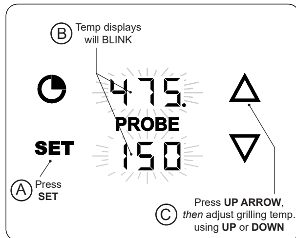
Fig. 35-1 Set grilling temp.
