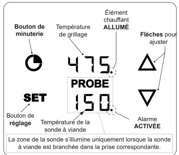
Fig. 38-1 Orientation (écran par défaut)
