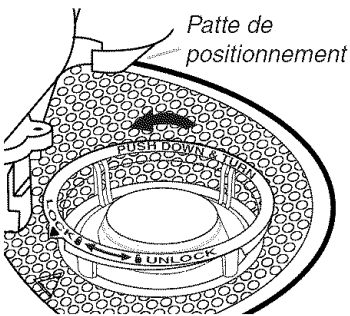
Dépose du filtre supérieur
