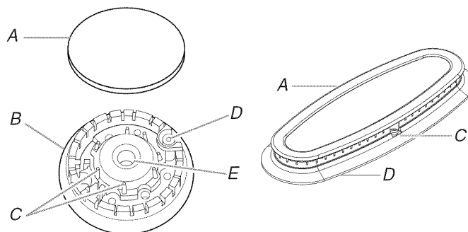
A. Burner cap B. Burner base
