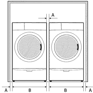
Área empotrada
