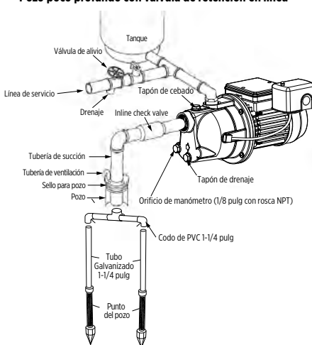
Pozo poco profundo con válvula de retención en línea
