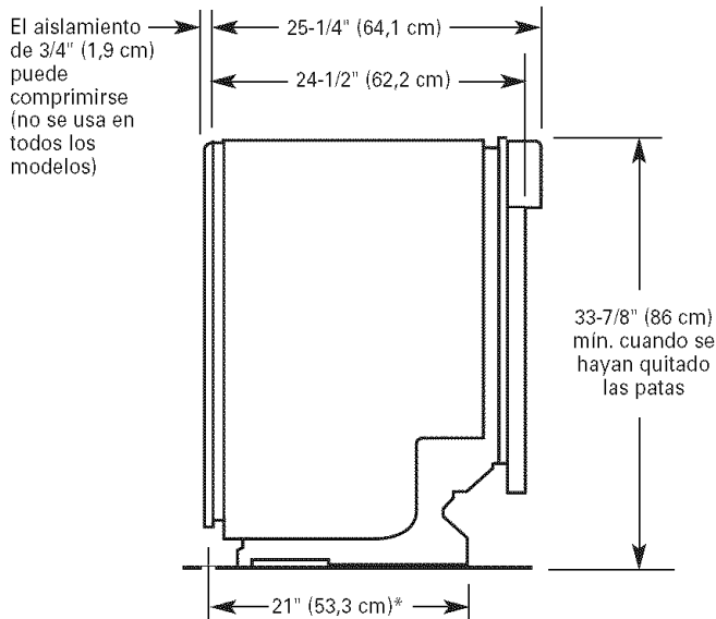
VISTA LATERAL
