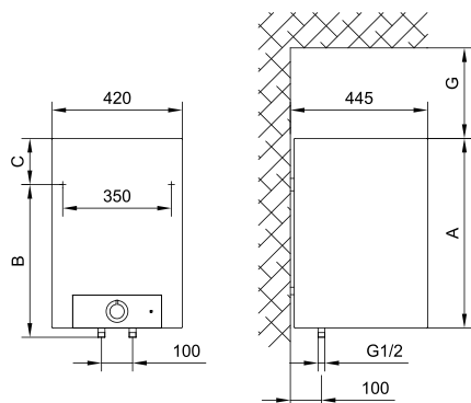
Priključne in montažne mere grelnika [mm]
