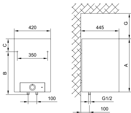
Priključne i montažne mjere grijalice [mm]
