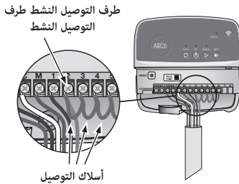
أسلاك التوصيل
