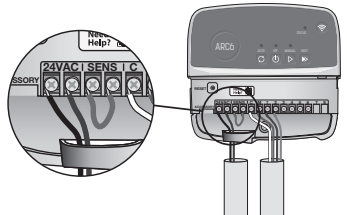
أسلاك التوصيل
