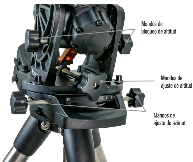
Figura 8 Regulación de alineación polar
