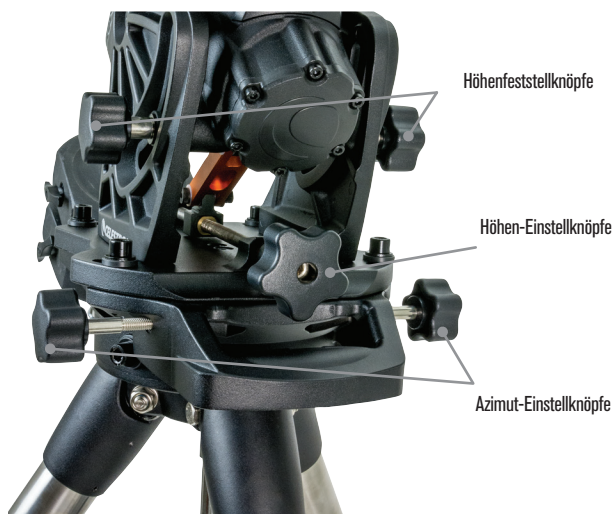
Abbildung 8 Polarausrichtungseinstellung
