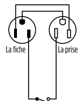
Interrupteur vertical avec une fiche superposé (« piggyback »)
