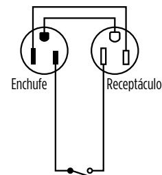
Interruptor vertical con un enchufe de combinación
