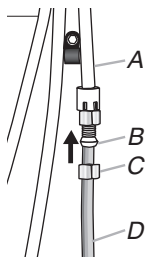
A. Canalisation d'eau en plastique B. Manchon C. Écrou à compression D. Tube en cuivre
