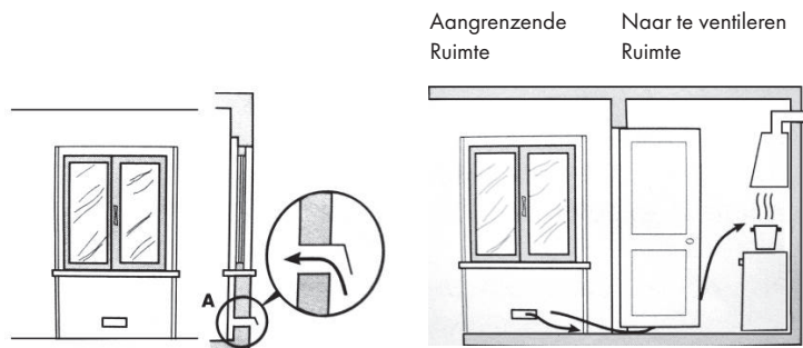
Voorbeeld van luchttoevoeropeningen voor de verbrandingslucht
