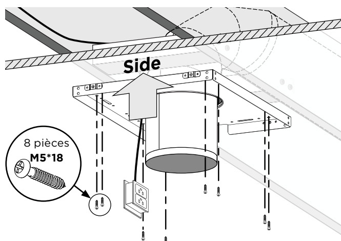
3.1 Événement latéral - Étage supérieur
