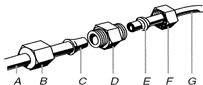
A. Tubería de agua del refrigerador D. Acoplamiento (adquirido) B. Tuerca (provista) E. Férula (adquirida) C. Bulbo F. Tuerca (adquirida) G. Línea de agua de la casa
