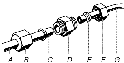
A. Conduit vers le réfrigérateur E. Virole (à acheter) B. Écrou (fourni) F. Écrou (à acheter) C. Renflement G. Canalisation d'eau du domicile D. Raccord (à acheter)
